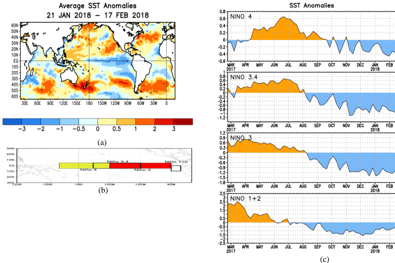
Figura 03 - (a) anomalia de temperatura da superfície do mar ( ^{\circ}\text{C} ) nos últimos 30 dias, (b) regiões de Niños e (c) evolução das anomalias da TSM ( ^{\circ}\text{C} ) nas regiões do Niño 4, Niño 3.4, Niño 3 e Niño 1+2 no Pacífico Equatorial. Fonte CPC/NCEP/NOAA, 2018
