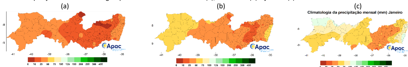
Figura 1 – Precipitação média climatológica para os meses de novembro (a), dezembro (b) e janeiro (c) em Pernambuco
