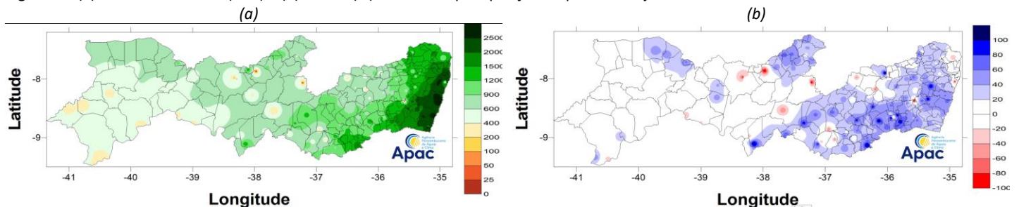
Figura 2 – (a) acumulado médio (mm) e (b) desvio (%) relativo da precipitação no período de janeiro a setembro de 2022.
