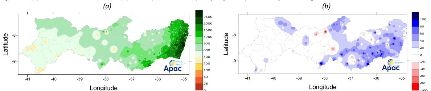
Figura 2 – (a) acumulado médio (mm) e (b) desvio (%) relativo da precipitação no período de janeiro a agosto de 2022.
