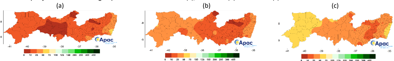
Figura 1 – Precipitação média climatológica para os meses de outubro (a), novembro (b) e dezembro (c) em Pernambuco
